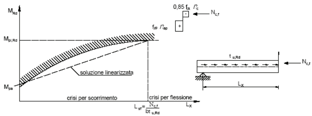
Figura C4.3.9 - Diagramma di interazione parziale calcestruzzo lamiera
