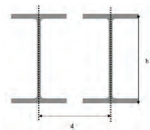
Figura C3.3.28 – Travi parallele
