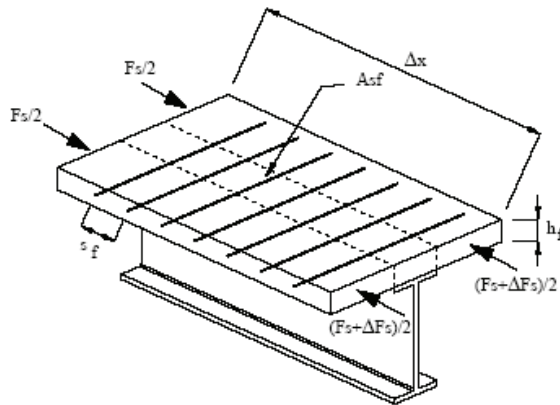
Figura C4.3.6. Distribuzione della sollecitazione di taglio longitudinale nella piattabanda di calcestruzzo
