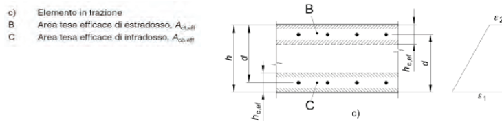
Figura C4.1.10- Area tesa efficace. Casi tipici
