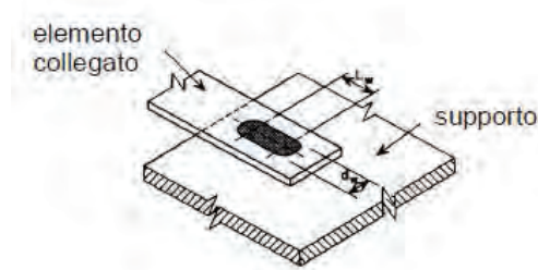
Figura C4.2.36 – Saldature oblunghe a bottone
