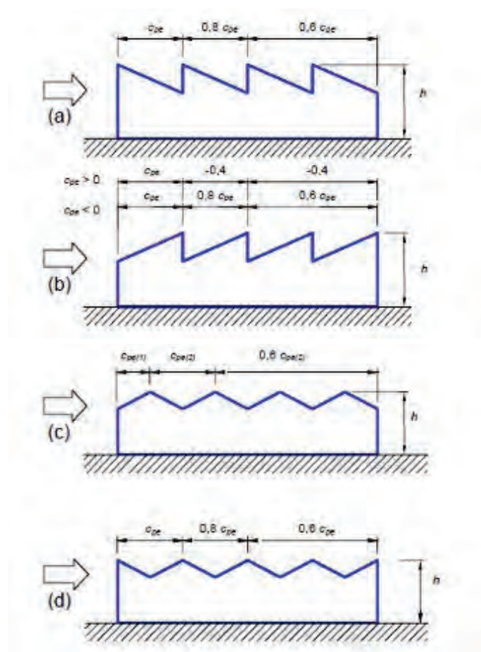
Figura C3.3.18 - Suddivisione delle coperture a falda multipla
