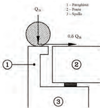
Figura C5.1.1 - Carichi da traffico su muri paraghiaia
