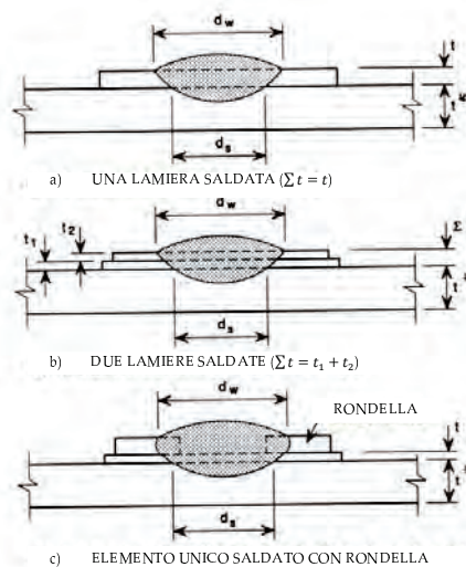
Figura C4.2.35 – Saldature a bottone
