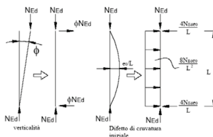
Figura C4.2.4 - Sistemi di forze equivalenti alle imperfezioni
