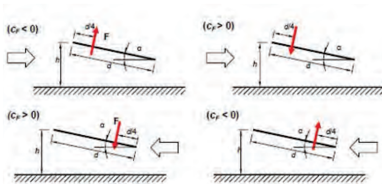
Tettoie a semplice falda: posizione del punto di applicazione della forza risultante in funzione della direzione di provenienza del vento e della direzione della forza
