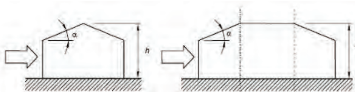
Figura C3.3.15 - Schema delle coperture a padiglione
