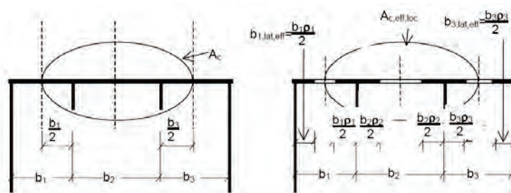
Figura C4.2.15 - Lastra irrigidita uniformemente compressa
