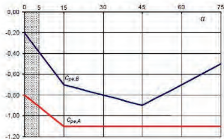
Figura C3.3.9 - Coefficienti di pressione per coperture a semplice falda: vento parallelo alla direzione del colmo
