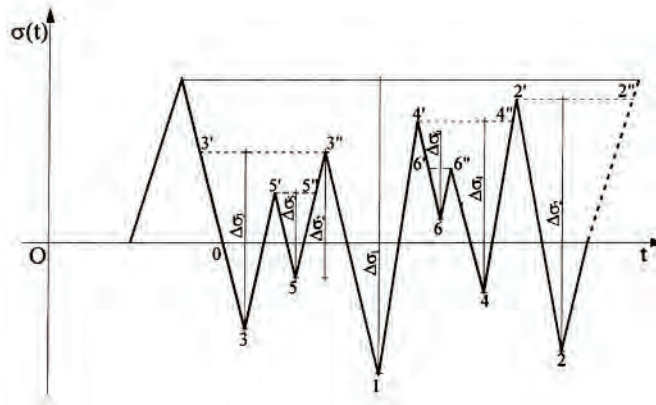
Figura C4.2.19 - Metodo del serbatoio
