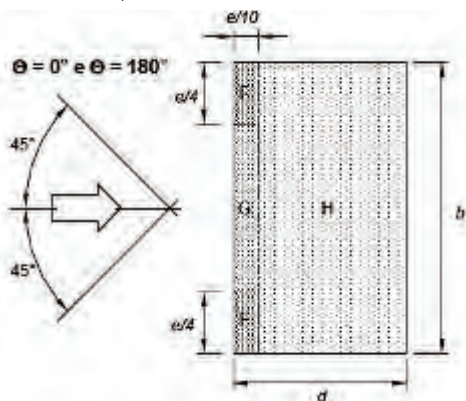
Vento ortogonale alla direzione del colmo
